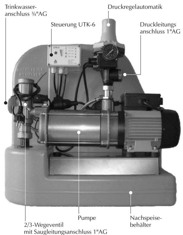
Abb. 4 Aufbau
