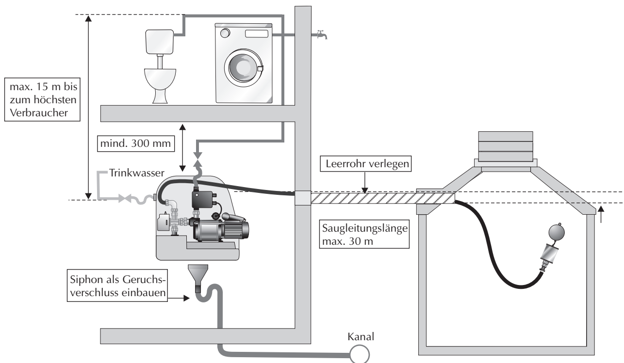
Abb. 8 Hydraulischer Anschluss der Box V60E
