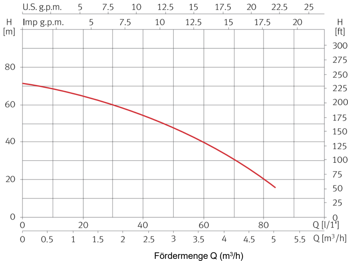
Diagramm 3.5.1 Kennliniendiagramm AMRES bei 2900 min -1
